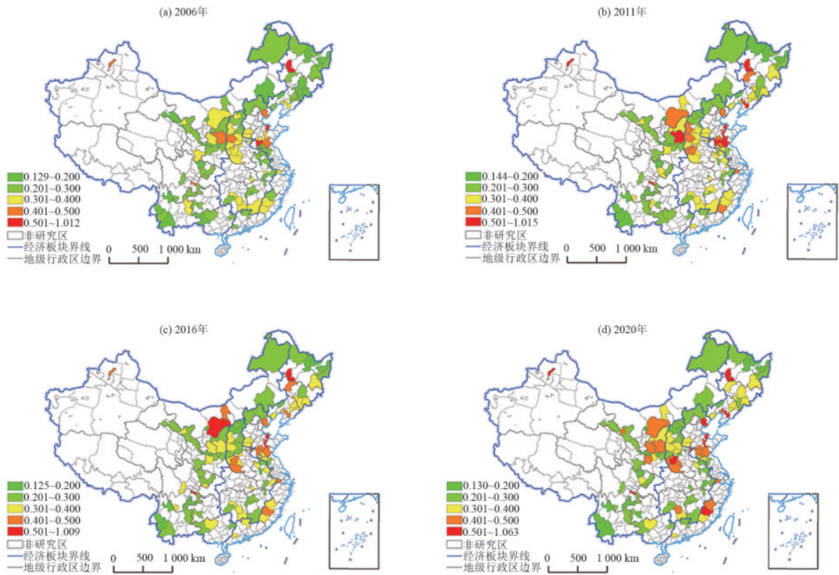
图 4 资源型城市土地绿色利用效率空间分布格局
