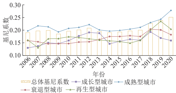
图 7 总体及不同成长阶段资源型城市土地绿色利用效率的差异变化趋势
