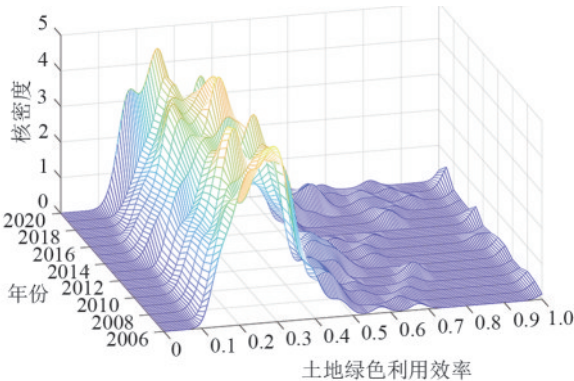
图 5 资源型城市总体核密度
