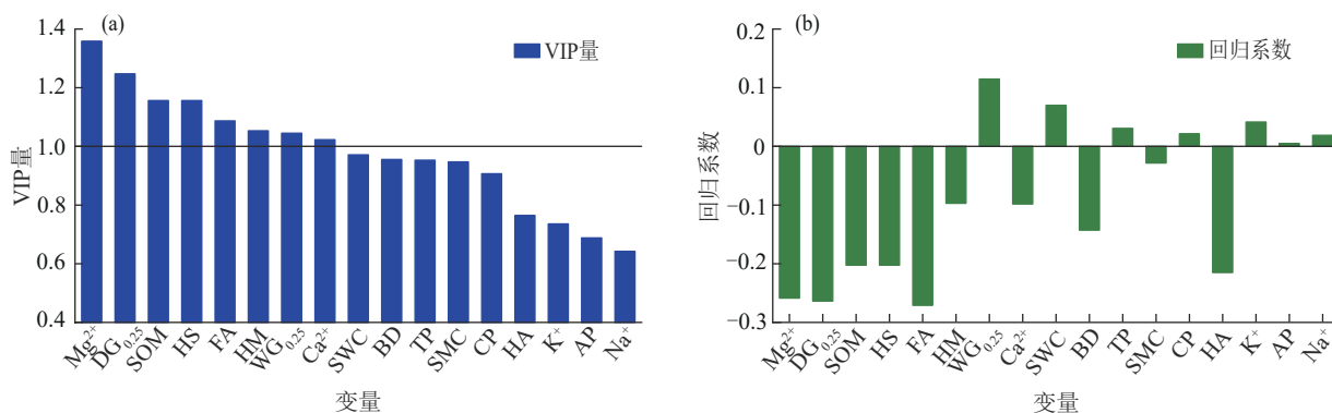
图3 K_d 偏最小二乘回归最优模型中土壤理化性质的变量投影重要性指标(VIP)和回归系数
