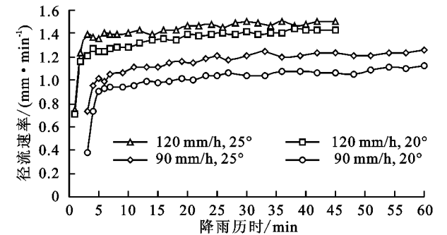
图 1 坡面径流速率随降雨历时的动态变化
