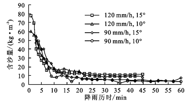
图 2 坡面径流含沙量随降雨历时的动态变化
