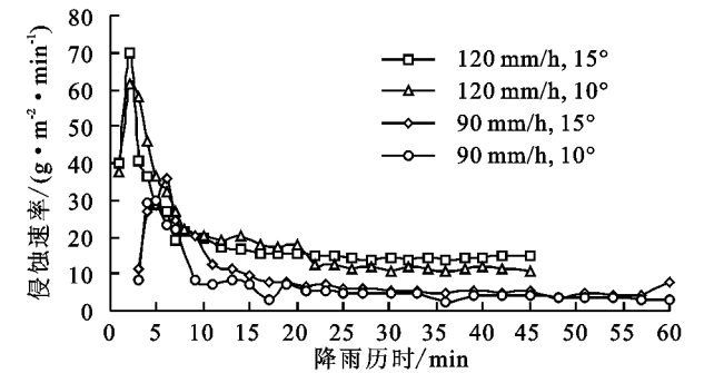
图 3 坡面侵蚀速率随降雨时的动态变化
