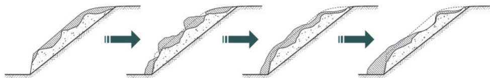
图9 火后泥石流初期的坡面泥石流演化模式
