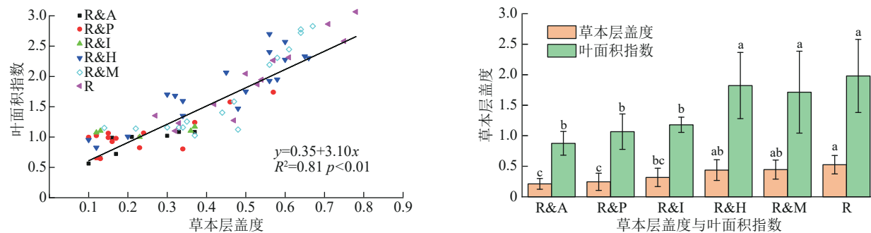
图 4 叶面积指数和草本层盖度
